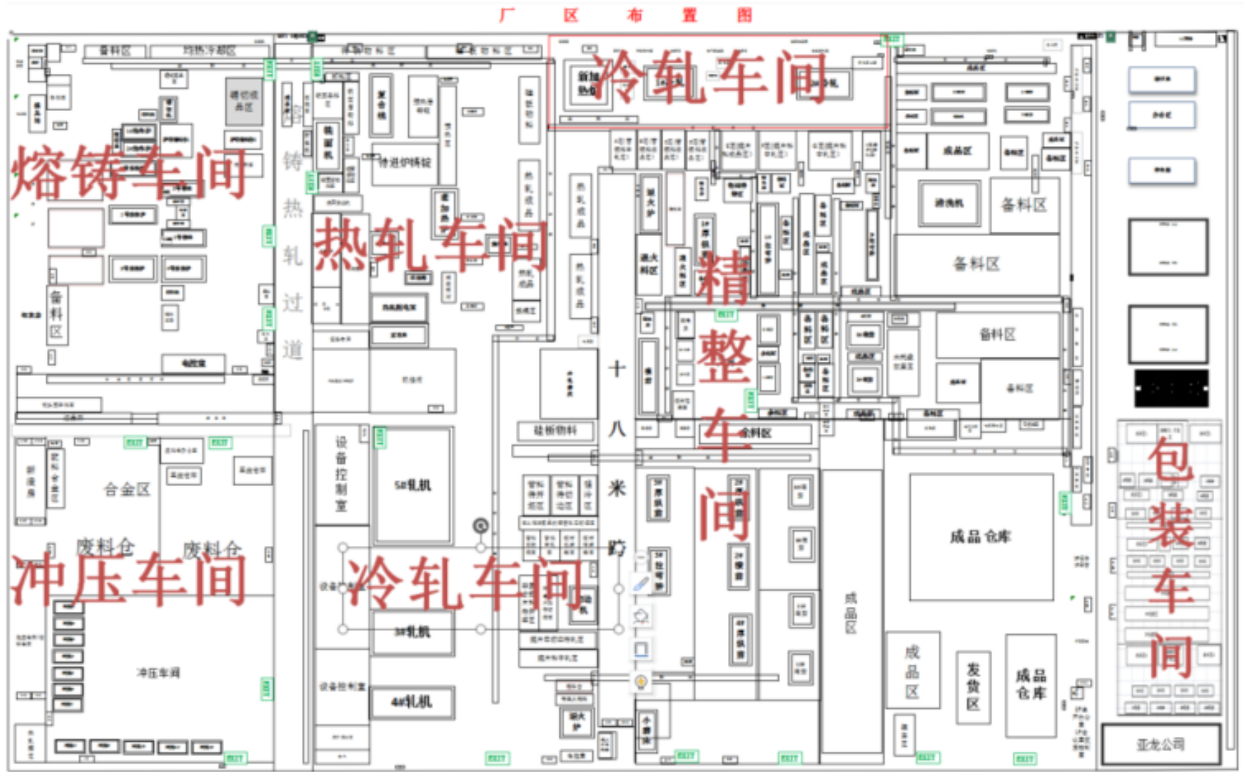
上海华峰铝业股份有限公司厂区布局平面图
